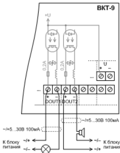
Рисунок 5.9 – Дискретные выходы
